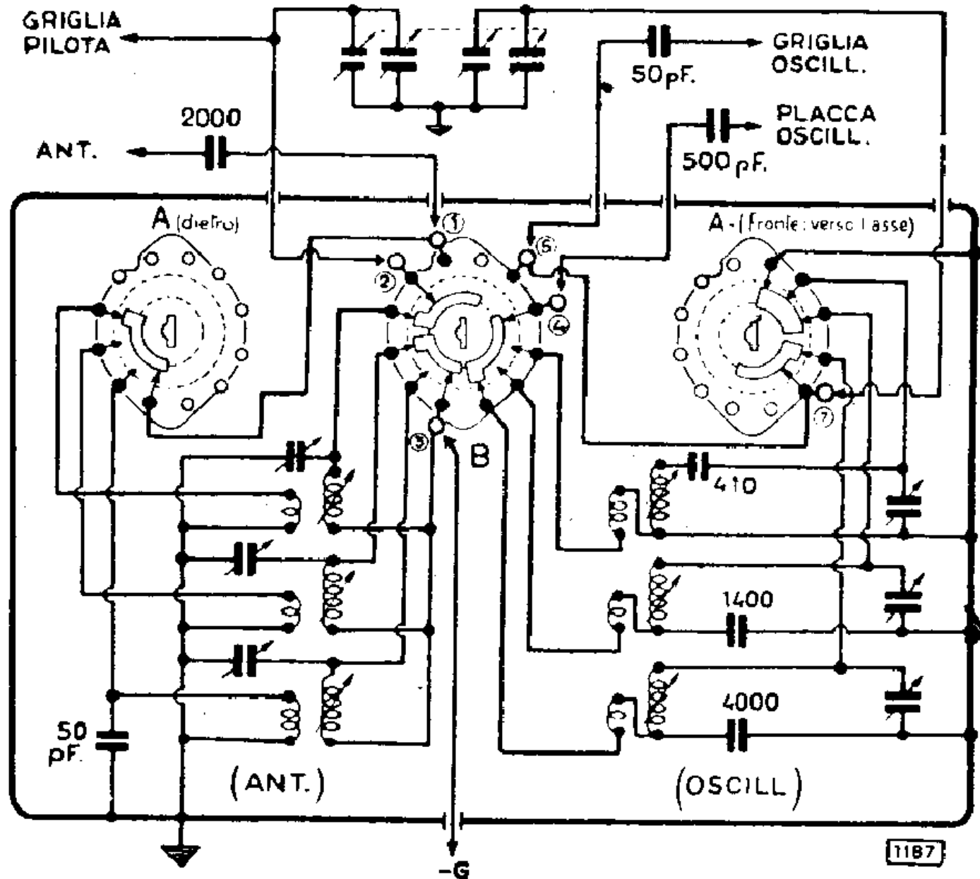
Commutatore visto di dietro, disegnato nella posizione onde più corte
